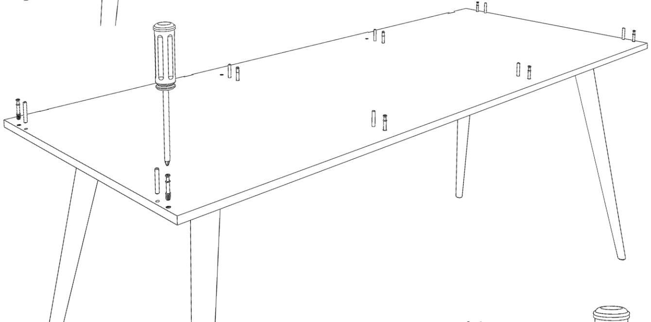
Корпус и ящики собираем на эксцентровые стяжки
